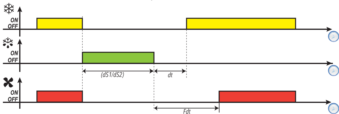
Abtauende mit Heizwiderständen durch Temperatur
